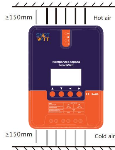
Рисунок 2-1. Установка и рассеивание тепла
