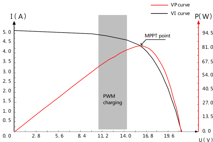
Рисунок 1-2. График выходных параметров солнечного модуля
