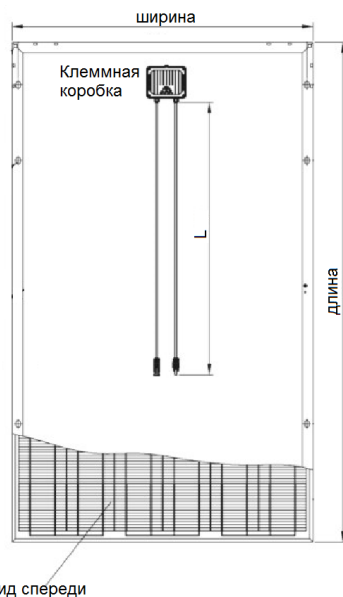
Рисунок 1 – схематическое изображение ФЭМ
